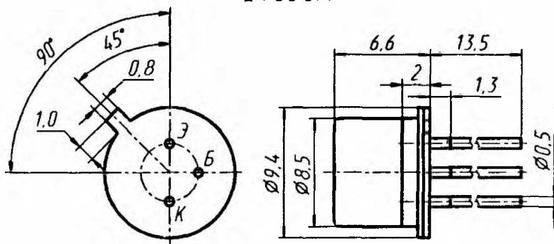
2Т638А
