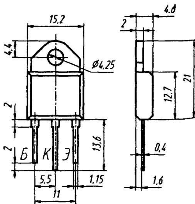
КТ819(А1-Г1)
