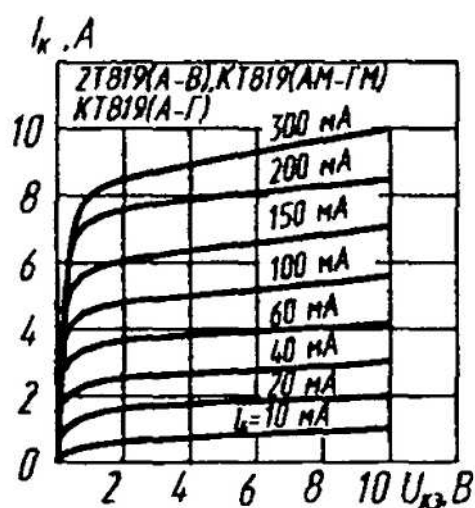
Выходные характеристики
